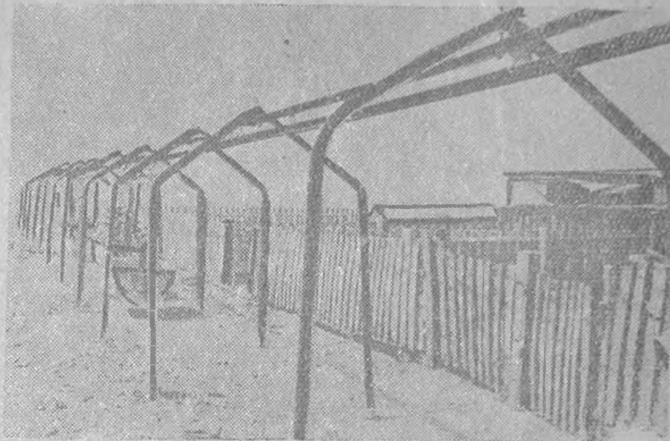
Западн района „Ленинец“ колхозд малд кбдлдж улсин кбдлмш амрудлгннд ик оньг бггдлжәнә. ЗУРГТ: Малин хашад тосхгдджджх подвесн хаалгь. Эн хаалгь утлан 270 метр.
