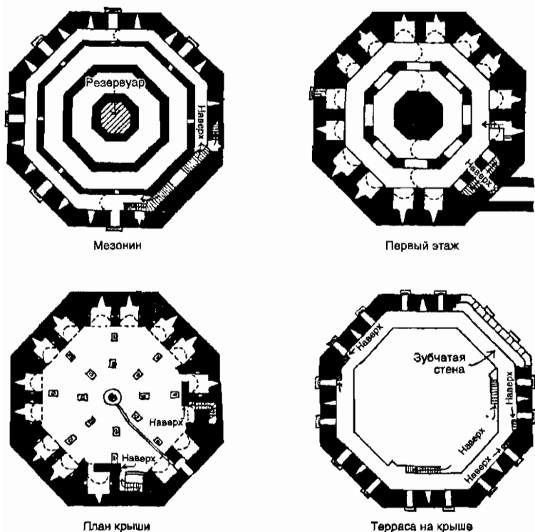
Рис. 206. Планы пола и крыши Кызыл Куле, Алай
