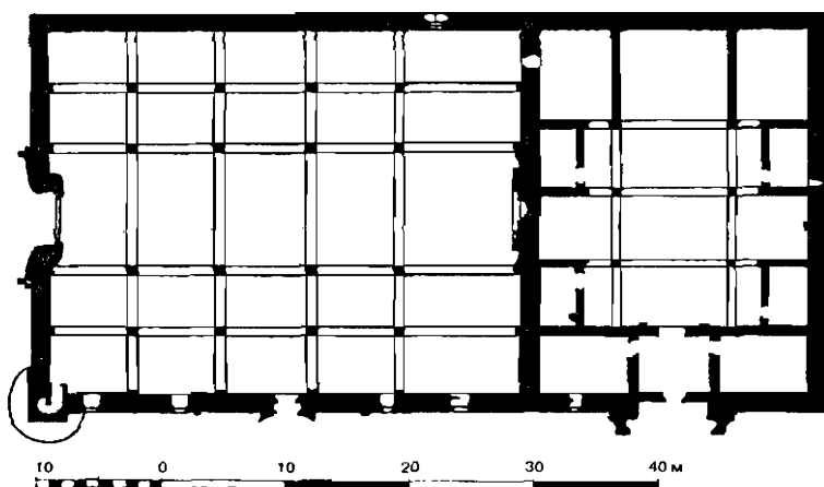
Рис. 16. План улу джами и больницы для душевнобольных в Дивриги, 1228 г.
