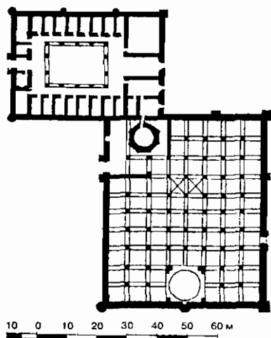
Рис. 10. План комплекса Мафери-хатун в Кайсери, 1237/38 г.: мечеть, мавзолей и медресе; бани до наших дней не сохранились
