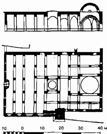
Рис. 14. Вертикальная проекция и план улу джами Кайсери; строительство мечети начато в 1135 г., завершено в 1205 г.
