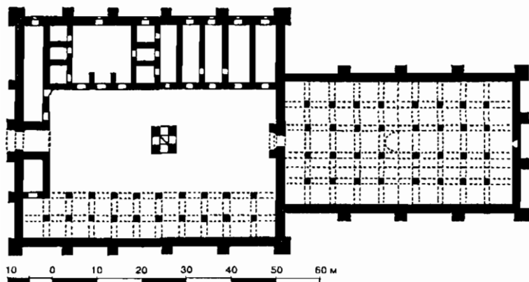
Рис. 8. План Султан-хана на дороге Конья—Аксарай, 1229 г.
