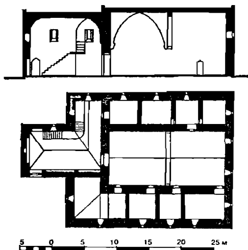
Рис. 5. Вертикальная проекция кешка Хайдар-бея
