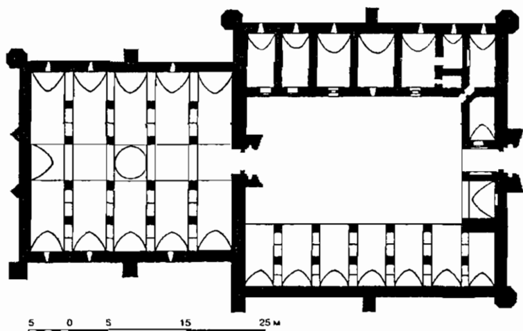
Рис. 19. План хана Сары на дороге Ургюп—Аванос, 1238 г.
