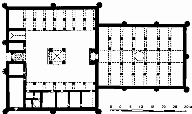
Рис. 15. План Султан-хана на дороге Кайсери—Сивас, 1230/31 г.
