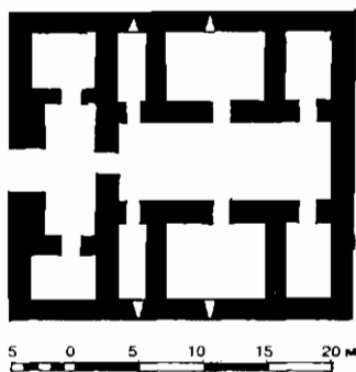
Рис. 26. План малого здания в Кубадабаде, 1235 г.
